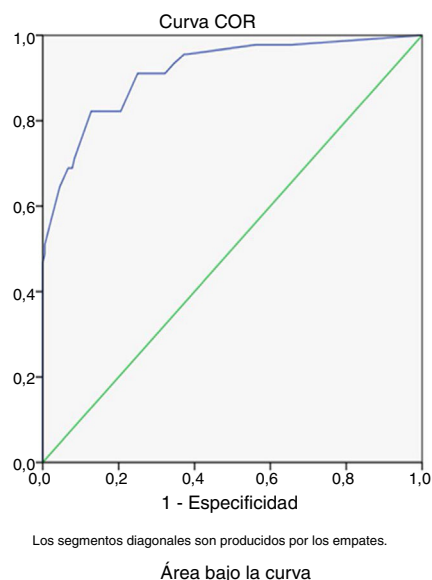
Variables resultado de contraste: probabilidad pronosticada
