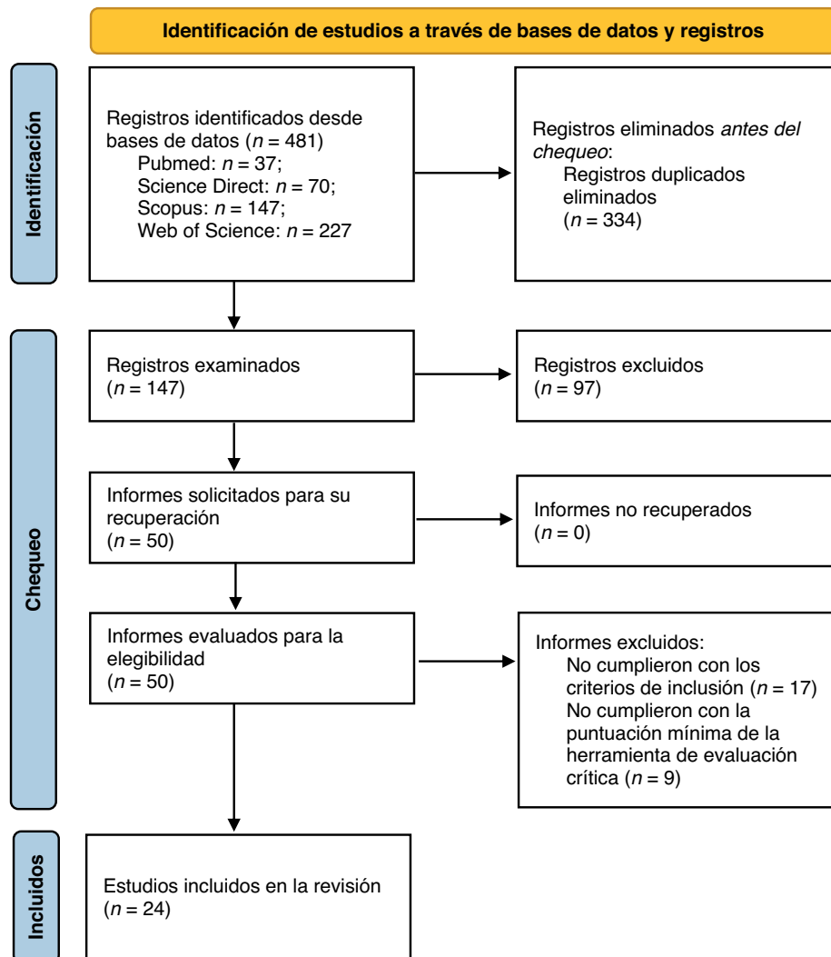
Figura 1 Diagrama PRISMA.
