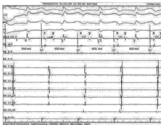
Figura 8. Dobles potenciales a lo largo de la línea de ablación. De arriba a abajo: derivaciones ECGs II, III, aVF, V 1 , electrogramas endocárdicos en el sitio de la línea de ablación (ABLd) y a lo largo del anillo tricuspídeo (RA-1-2 a RA-19-20) y seno coronario. Estimulación a un ciclo S1S1 600 ms. Dobles potenciales (XY) ampliamente separados (130 ms) sobre el catéter de ablación (ABLd), confirmando el bloqueo bidireccional del istmo.
