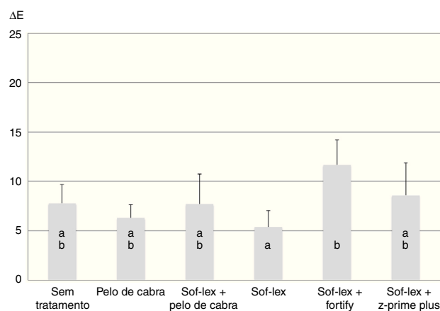
Figura 3 – Valores médios de ΔE e desvio padrão de acordo com a técnica de acabamento para o Protemp 4 com um período de exposição de 24 horas. Colunas com letras iguais representam valores médios de ΔE estatisticamente semelhantes ( p \geq 0,05 ).
