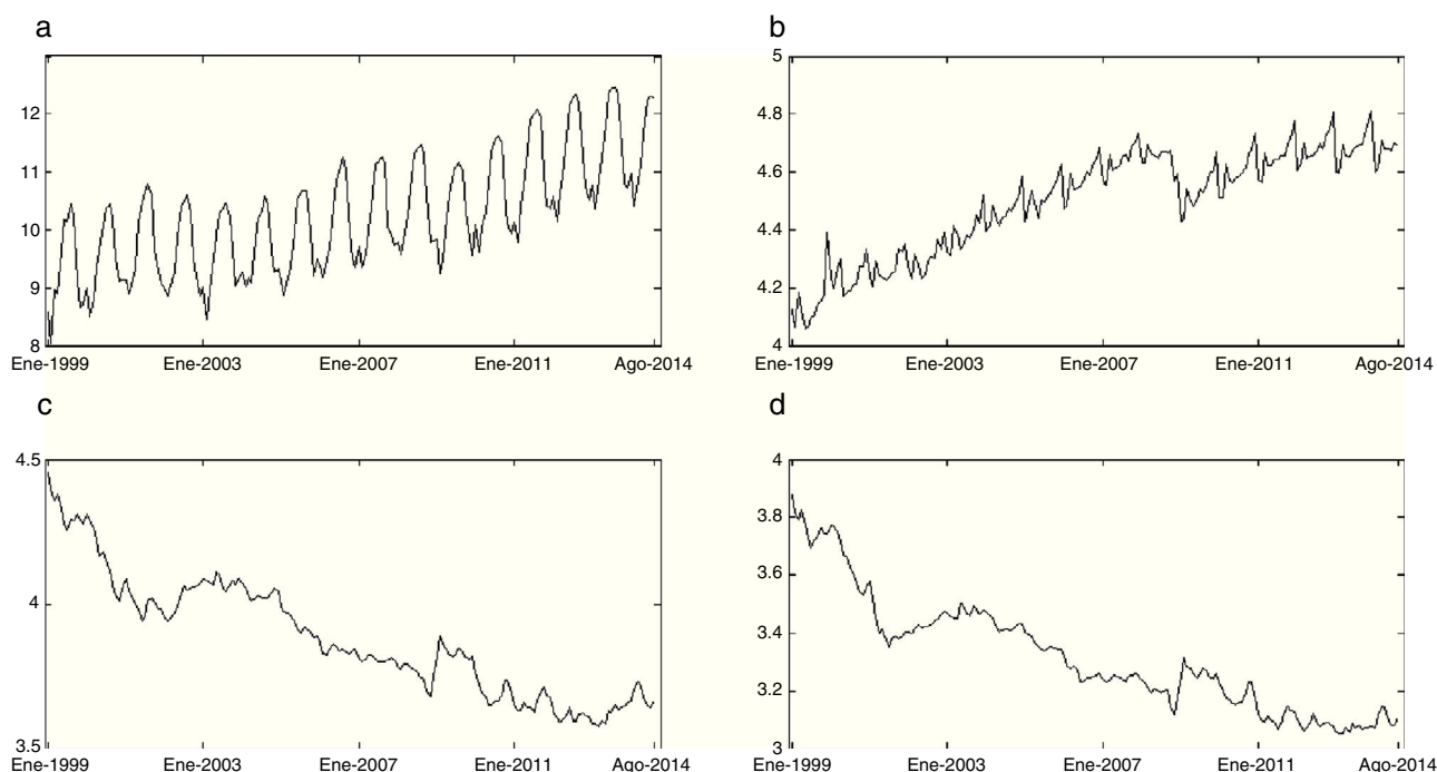
Figura 1 Evolución temporal de las llegadas de turistas rusos y de las variables socioeconómicas. (a) Logaritmo de las llegadas de turistas rusos. (b) Logaritmo del Índice de Producción Industrial (IPI) ruso (R). (c) Logaritmo del indicador del diferencial del coste real entre España y Rusia (P). (d) Logaritmo del indicador del diferencial del coste real entre Rusia y otros destinos turísticos (PS).
