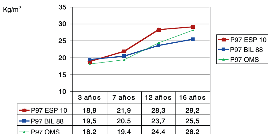
Figura 7 Comparación de los valores de los percentiles 50 y 97 del índice de masa corporal para mujeres entre el estudio transversal español 2010, el estudio de Bilbao 1988 y el estudio de la OMS, a las edades de 4, 10 y 18 años (datos obtenidos de Hernández et al 11 1988, WHO 40 2006 y Carrascosa et al 22 2010).
